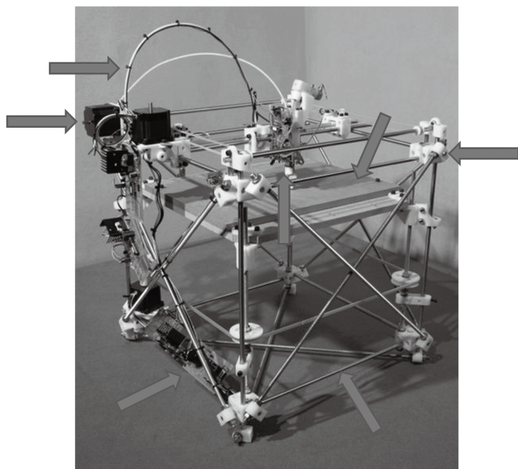
圖3.2. RepRap印表機
