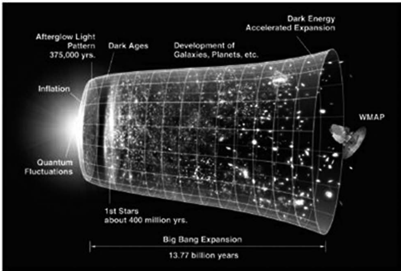
圖1.3. 宇宙在其數十億年歷史中發展和膨脹的圖示。
